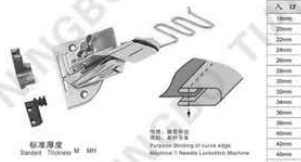
TL-120 K10 平头直角包边器 Right Angle Book Binder
